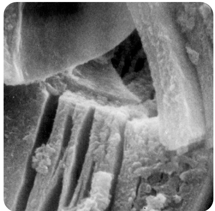
Ílový minerál
