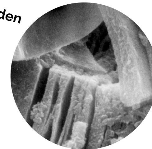
minerale argiloase
